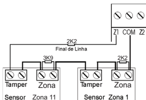
Ligação para sensores que possuem tamper
