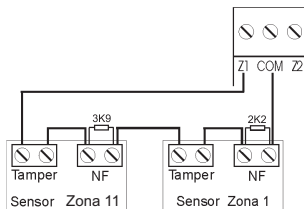
Ligação para sensores que possuem tamper
