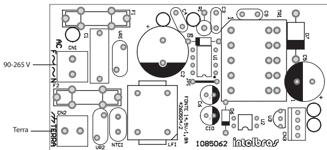
Fonte AC
