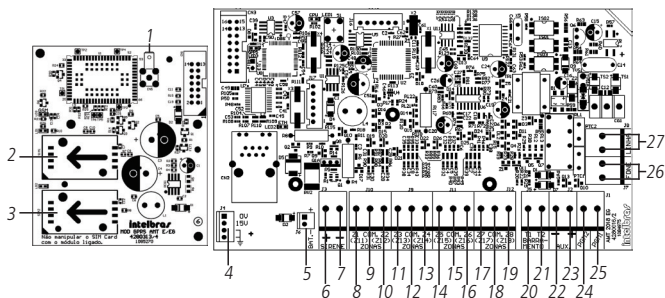
Placa GPRS
