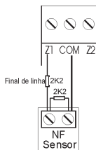
Ligação para sensores sem tamper
